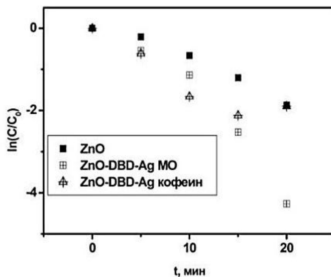
Рисунок 1 – Сравнение фотокаталитической активности допированных наночастицами серебра фотокатализаторов на основе оксида цинка в реакциях фотодегradации МО и кофеина: кинетика реакции фотодегradации МО (кофеина) определена по измерению оптической плотности на \lambda = 465 (272) нм
