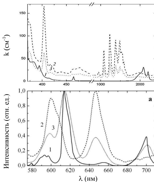
Рисунок 1 – Спектры поглощения (б) и люминесценции (а) однолегированных европием (1) и самарием (2) и солегированных этими элементами (3) теллуритно-вольфраматных стёкол. \lambda_{\text{в}}, \text{nm} : 397 (1а, 2а) и 480 (3а)
