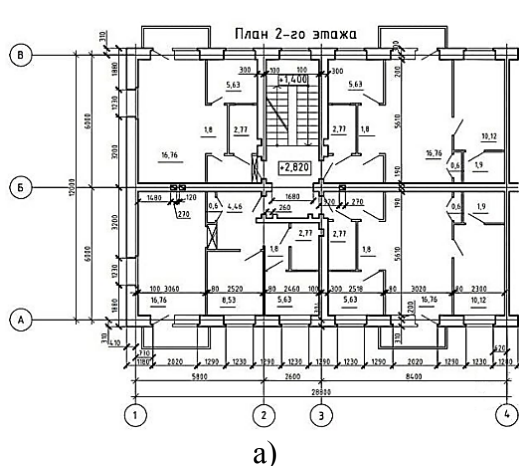
Рисунок 1 – а – план этажа; б – архитектурная 3D-визуализация в системе Autodesk 3ds Max
