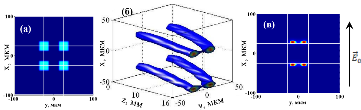
а – входное расположение пучков; б – трехмерная модель распределения светового поля по толщине кристалла; в – распределение светового поля на выходе из кристалла
