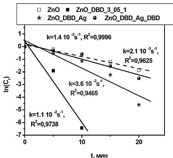
Рисунок 1 – Изменение значений логарифма относительной концентрации ( \ln C_t ) метилового оранжевого под действием УФ излучения в присутствии фотокатализаторов на основе ZnO
