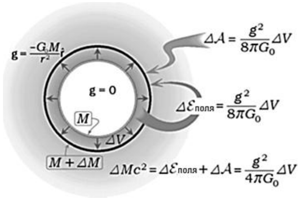
Рисунок 2 – Учет в энергетическом балансе увеличения энергии покоя гравитирующей сферической оболочки, расширяющейся под действием внешних сил в собственном поле, позволяет доказать положительную определенность плотности энергии поля Ньютона
