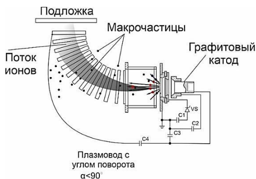
Рисунок 1 – Импульсный источник углеродной плазмы со свободновисящим фильтром (угол поворота потока на 90 градусов)
