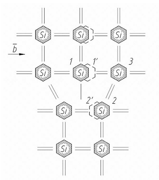
Рисунок 1 – Модель краевой дислокации для кремния
