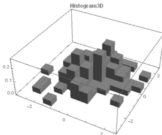
Рисунок 2 – Трехмерная гистограмма выборки data2
