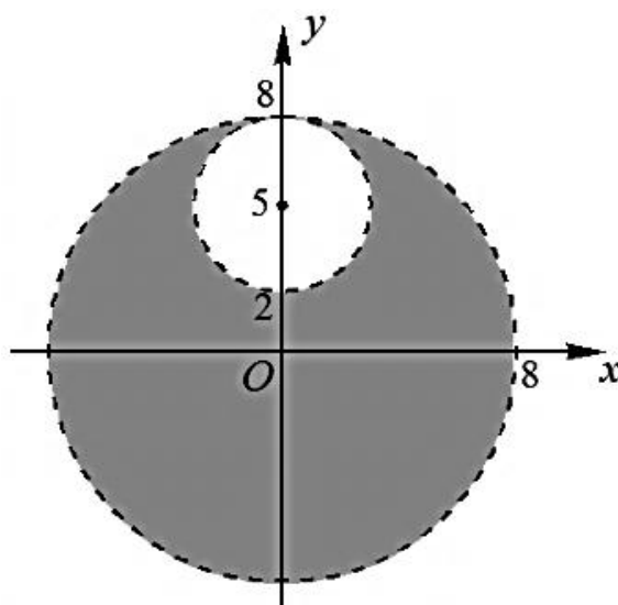
Рисунок 2 – Геометрическая интерпретация второй системы неравенств
