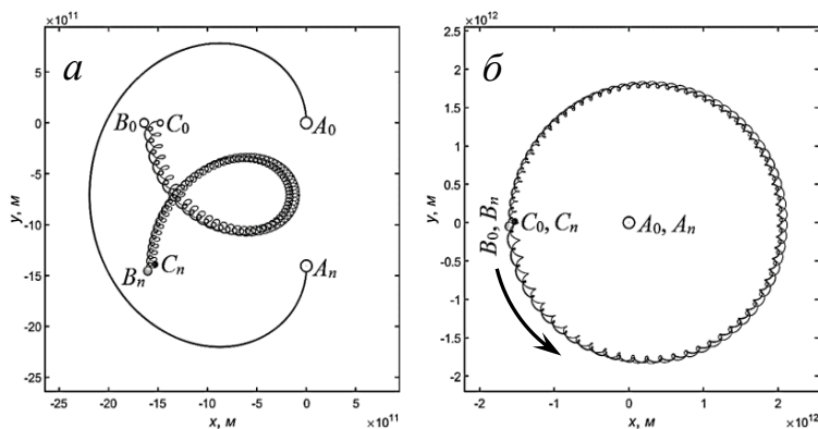
Рисунок 1 – Моделирование движения компонент тройной звездной системы HD 188753: а – относительно Солнечной системы, б – относительно компоненты HD 188753 A
