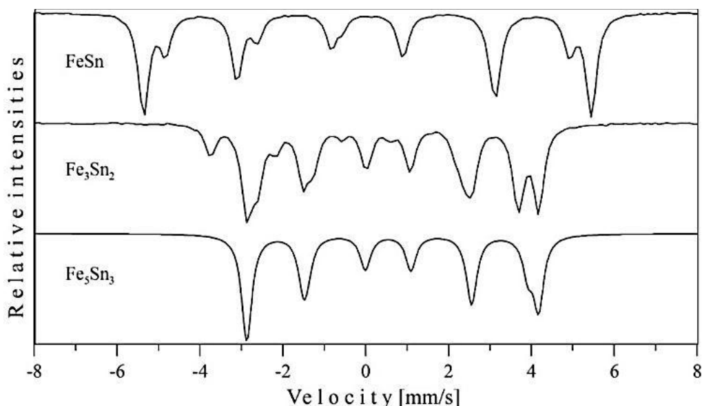
Рисунок 2 – Модельные спектры различных фаз бинарной системы Fe-Sn
