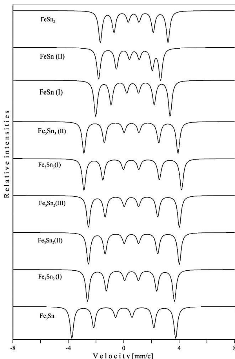
Рисунок 1 – Моделированные мессбауэровские спектры ядер ^{57}\text{Fe} в различных позициях интерметаллических фаз бинарной системы Fe-Sn
